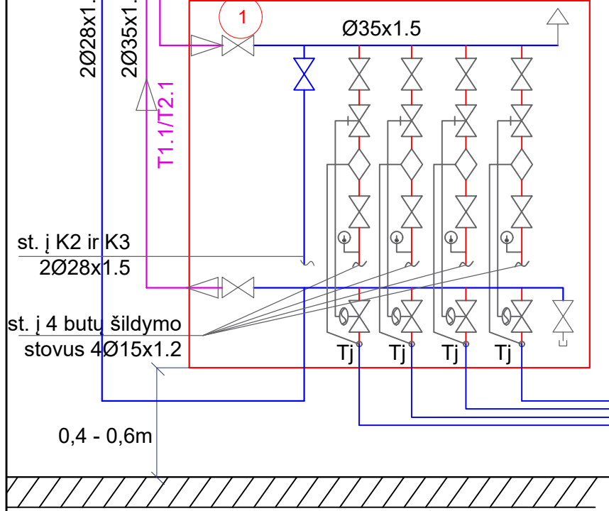
SCH.NR.1 ŠILDYMO KOLEKTORIUS SU APSKAITA VIRŠTINKINĖJE SPINELĖJE (PUSRŪSYJE) K1 5 ŠAKŲ (t.t. 4 ŠAKOS SU APSKAITA)
